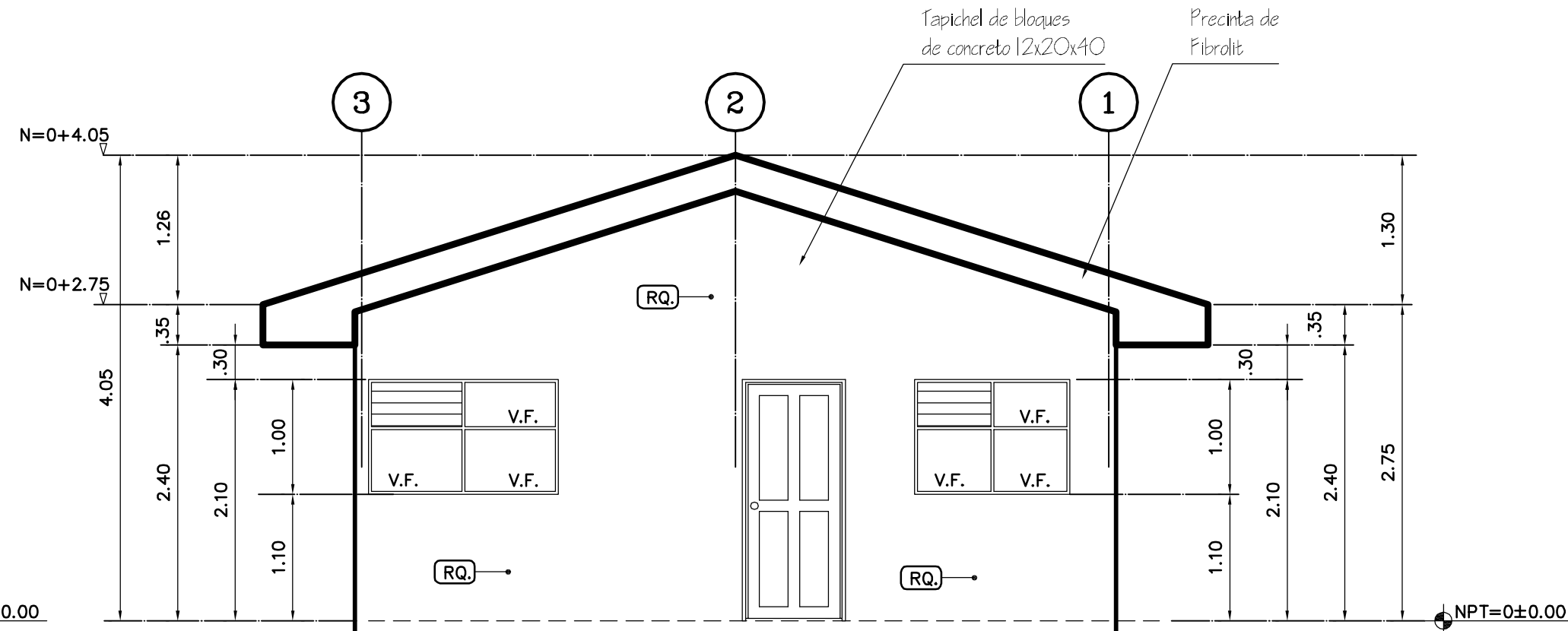
ELEVACION POSTERIOR.
