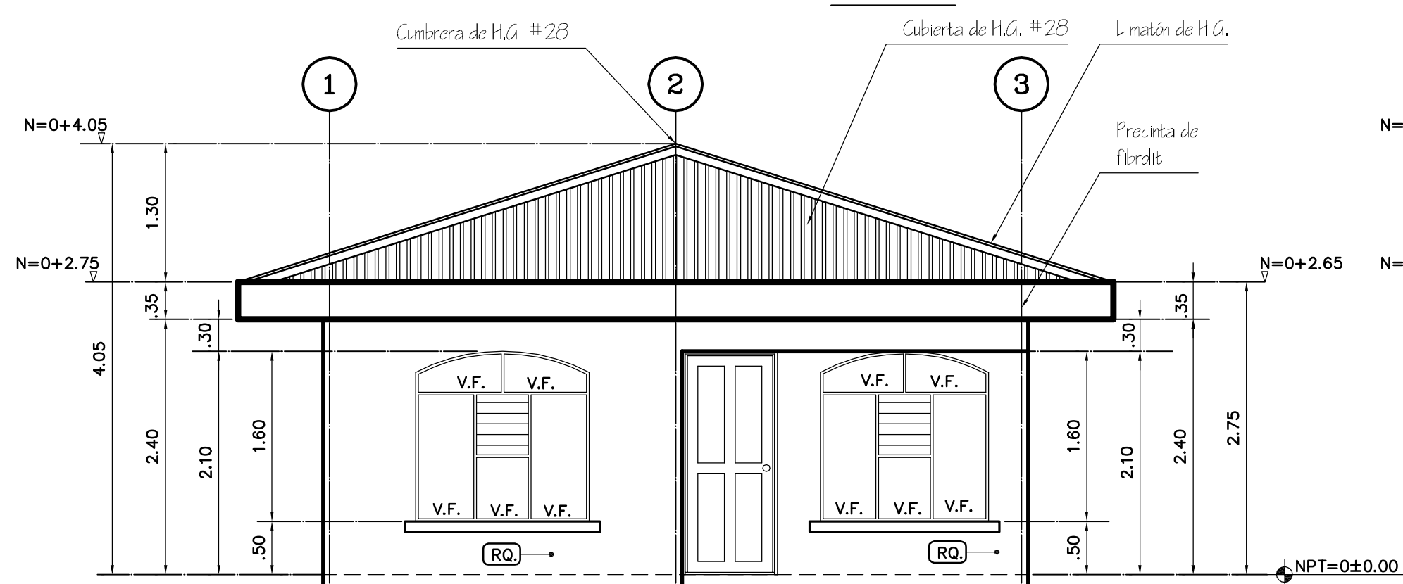
ELEVACION FRONTAL
