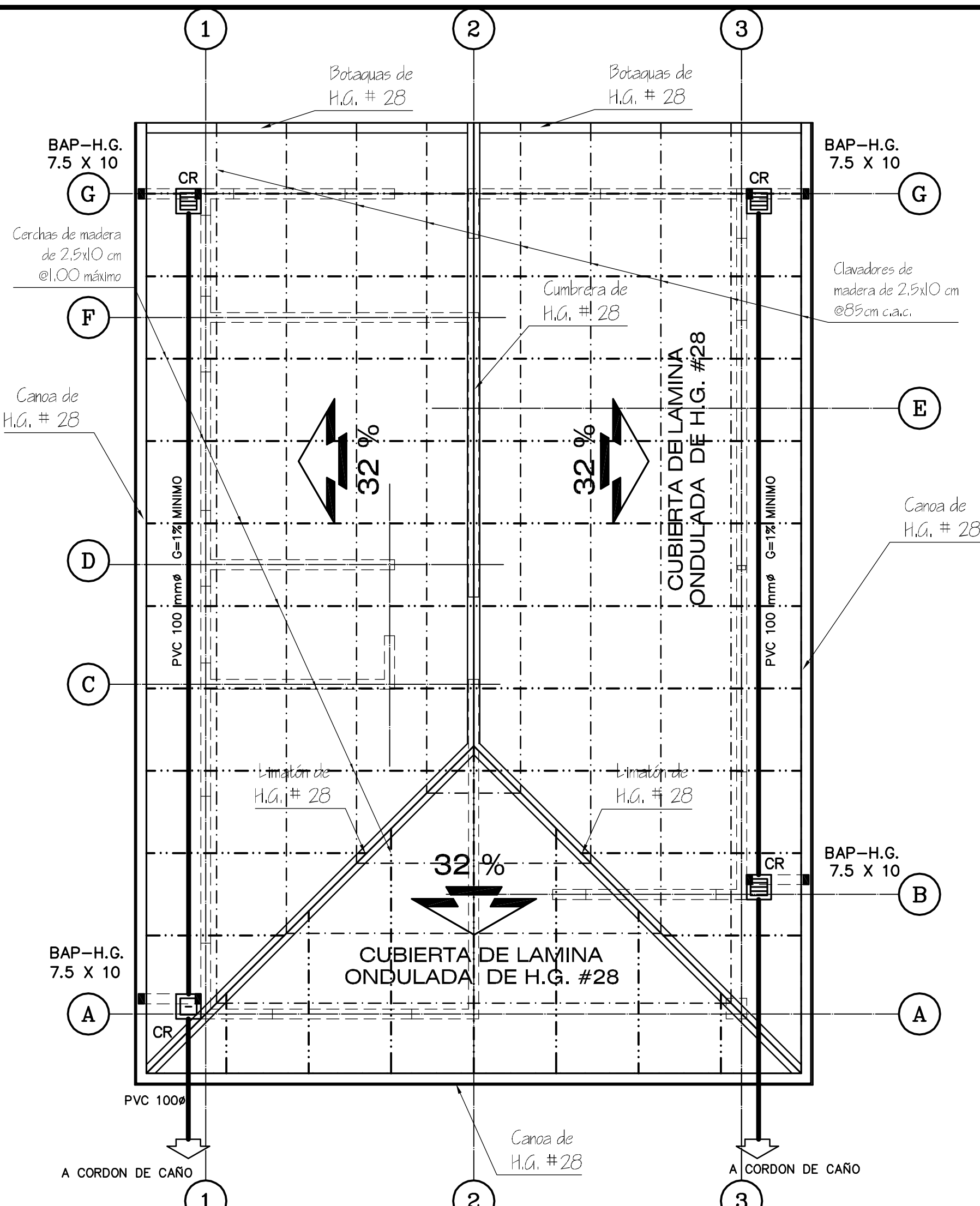
PLANTA DE TECHOS Y PLUVIALES
